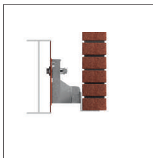
Fixation à une poutelle métallique
