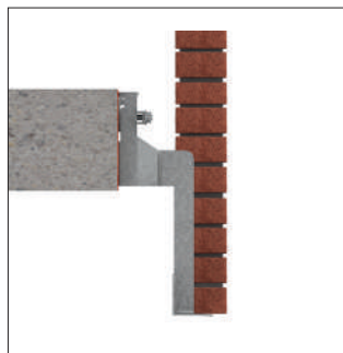
Avec latte devant volets roulant ou système de ventilation
